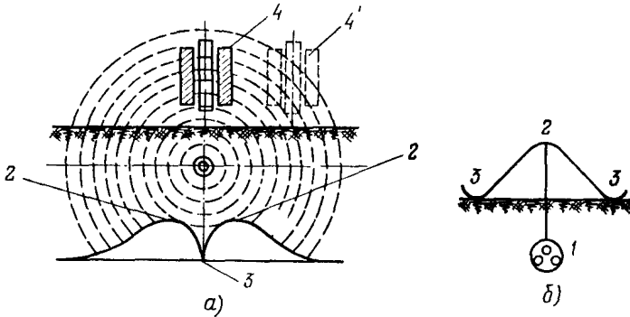
Рис. П9.1. Характер изменения звука при удалении рамки вправо или влево от линии прохождения кабеля:
