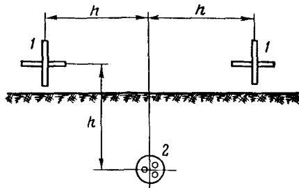
Рис. П9.2. Определение глубины заложения кабельной линии в земле индукционным методом:
